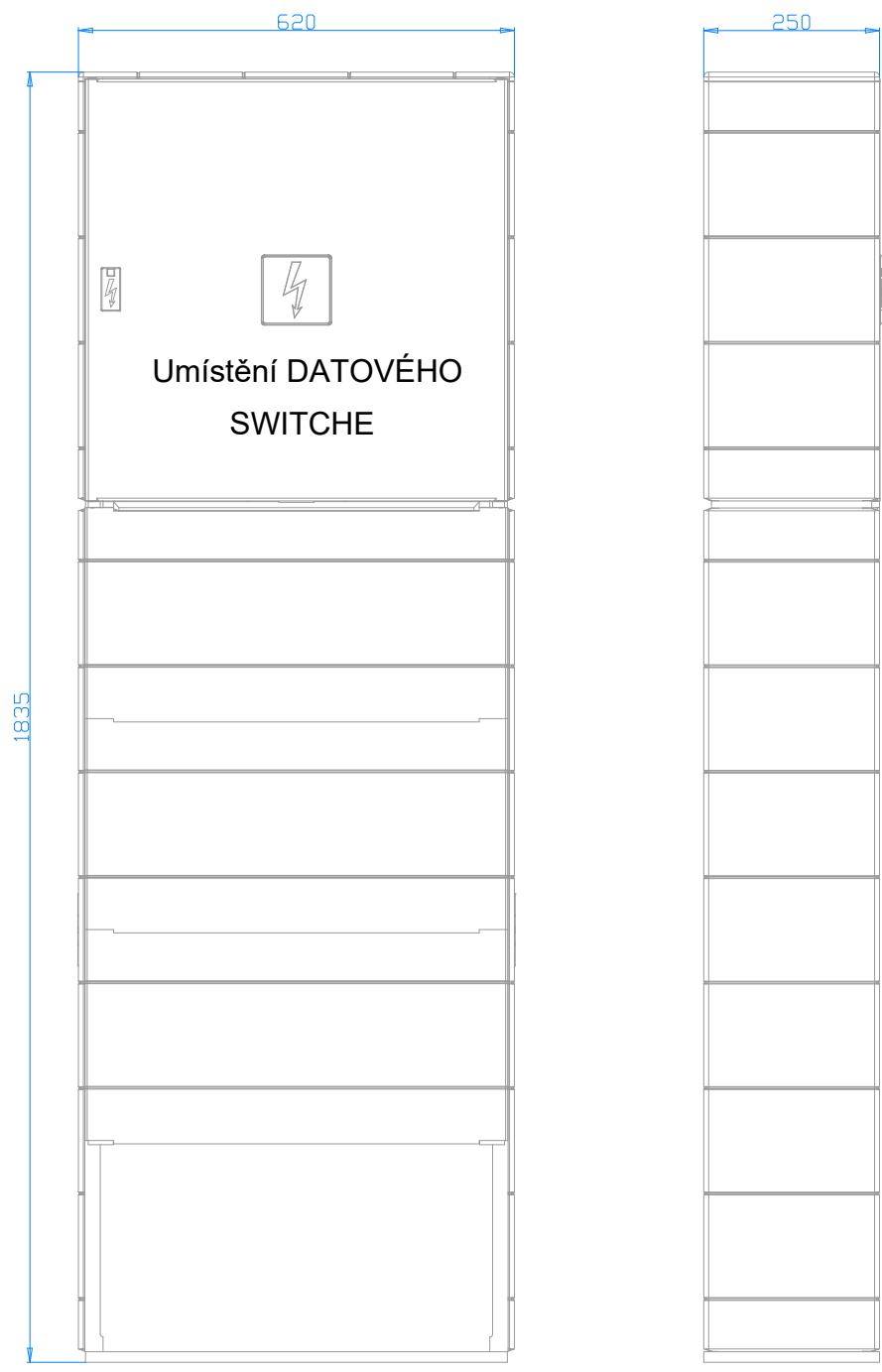
Prázdná skříň v pilířku, výrobce DCK HOLOUBKOV, IP44
