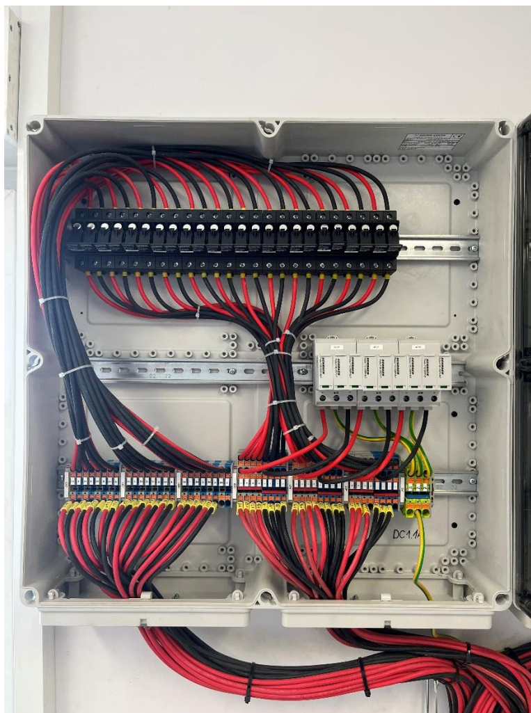
Obrázek č. 4 – RFVE – DC1.2a
