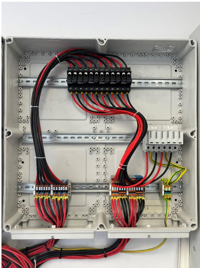
Obrázek č. 5 – RFVE – DC1b
