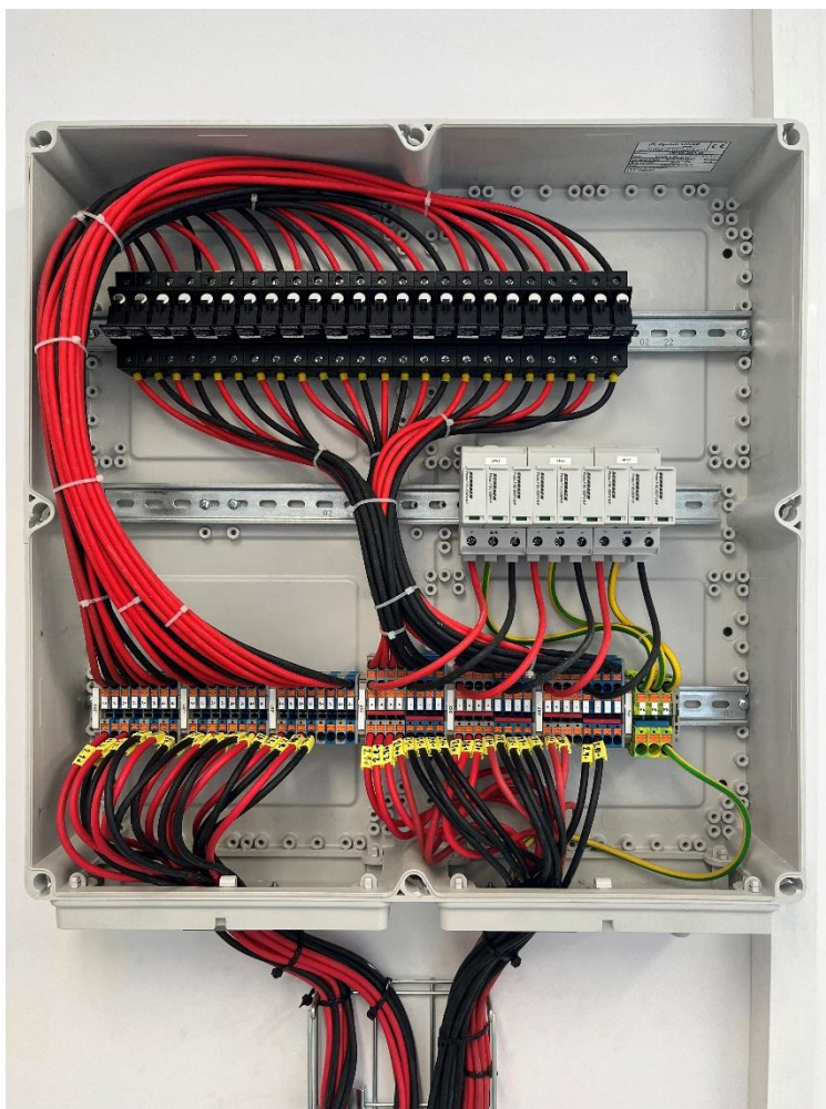
Obrázek č. 3 – RFVE – DC1.1a
