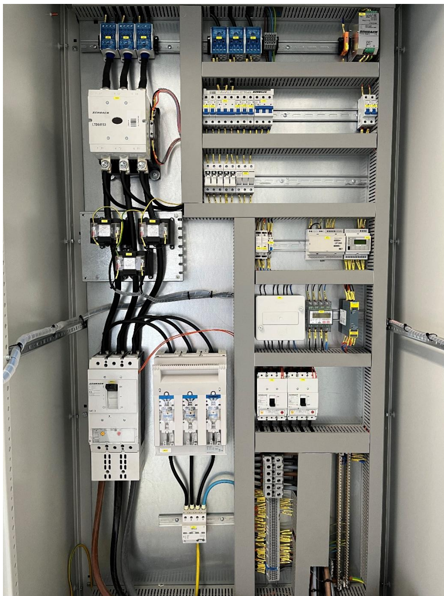
Obrázek č. 8 – Rozvaděč RFVE – AC1a
