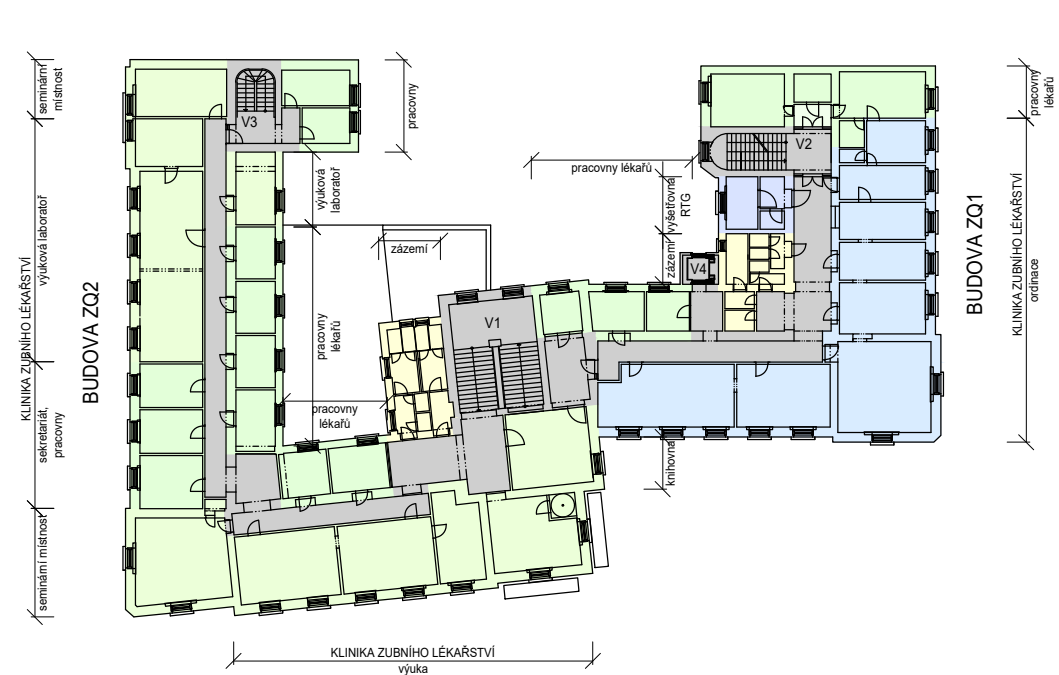
BUDOVA ZQ - 3.NP
