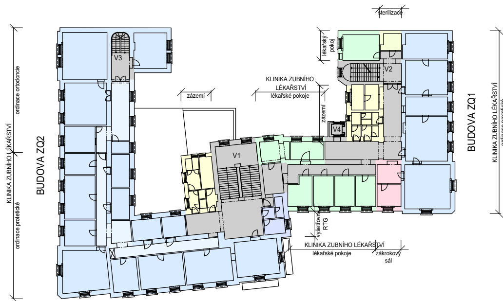
BUDOVA ZQ - 2.NP
