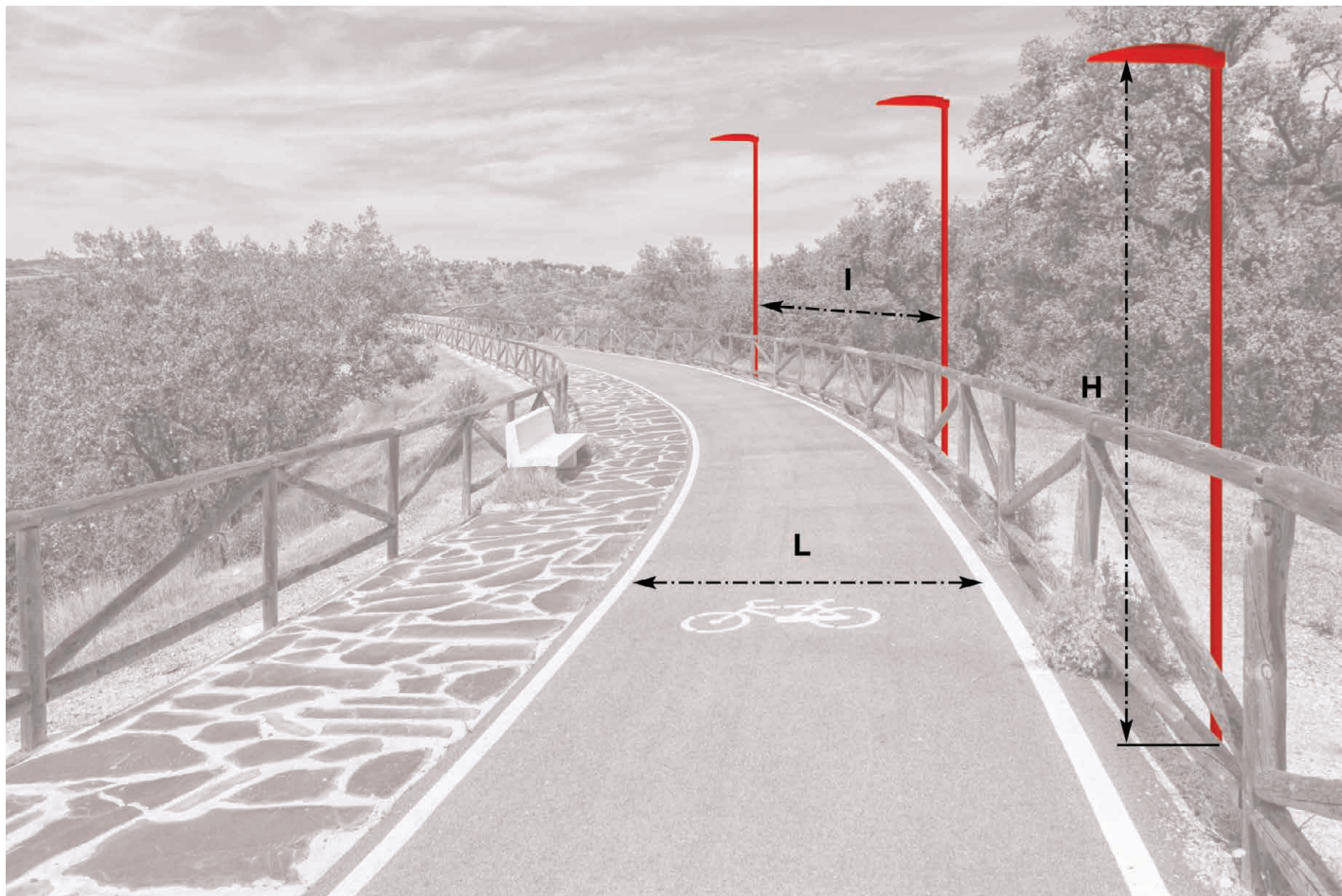
Aplikace osvětlení pro pěší a cyklisty podle ČSN EN 13201-2
