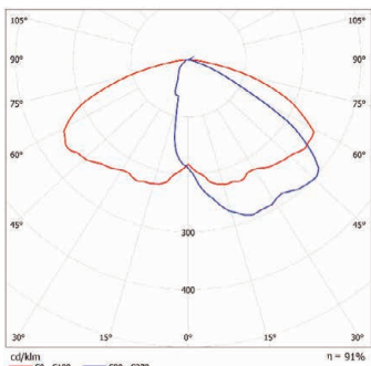
B) Optika městská / mimoměstská podélná
