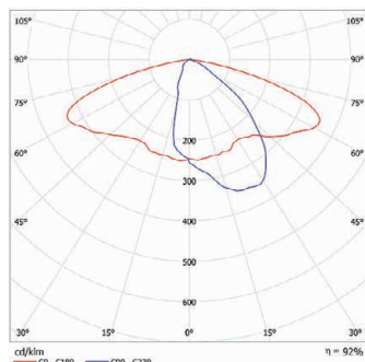
A) Optika pouliční městská / mimoměstská
