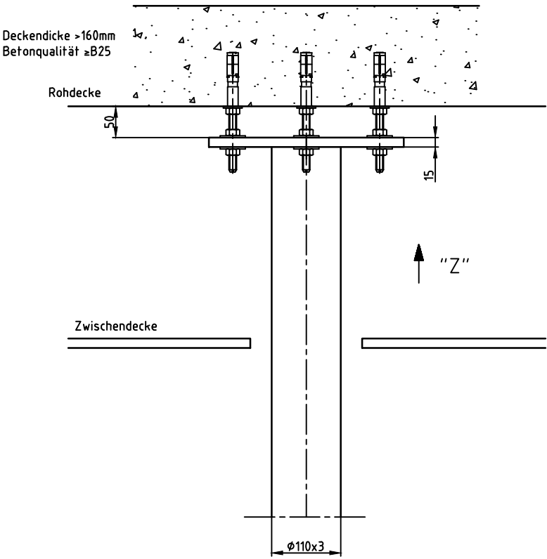
Ansicht "Y" M1:5 Vormontage Ponta-Deckenrohr
