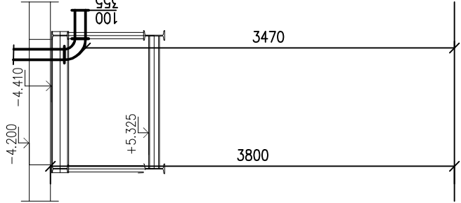
POHLED P2
