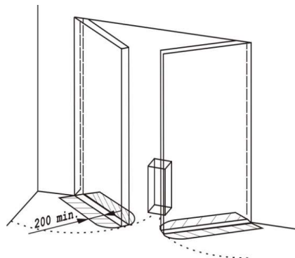
Obrázek C.5 – Dvoukřídlové kývavé dveře
