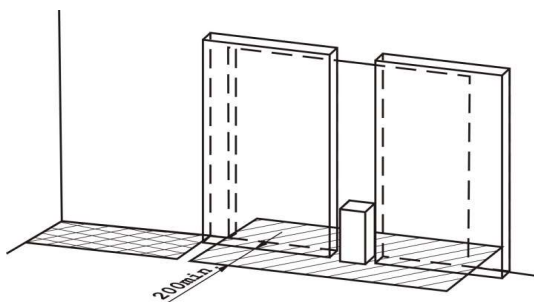
Obrázek C.2 – Jednokřídlové posuvné dveře
