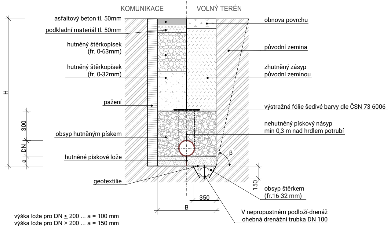
Šířka rýhy v závislosti na největším průměru potrubí
