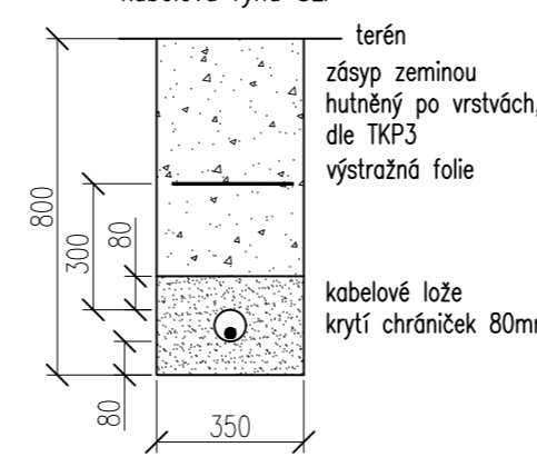
C VOLNÝ TERÉN, CHODNÍK kabelová rýha SLP
