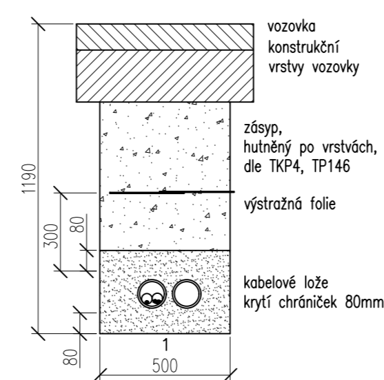
B POUŽÍDĚNÁ PLOCHA, KOMUNIKACE překop, kabelová rýha SLP
