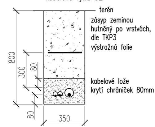
A VOLNÝ TERÉN, CHODNÍK kabelová rýha SLP
