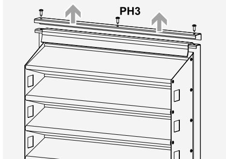
Obrázek 1 – uvolnění svěrných lišt
