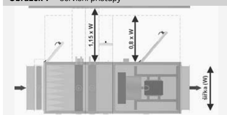
Obrázek 7 – servisní přístupy
