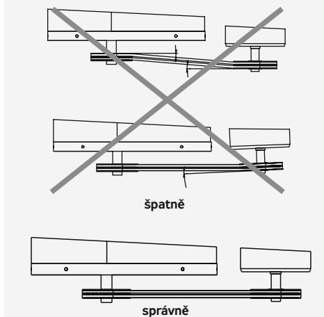
Obrázek 25 – srovnání řemenic
