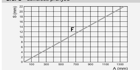
Graf 1 – závislosti průhybu
