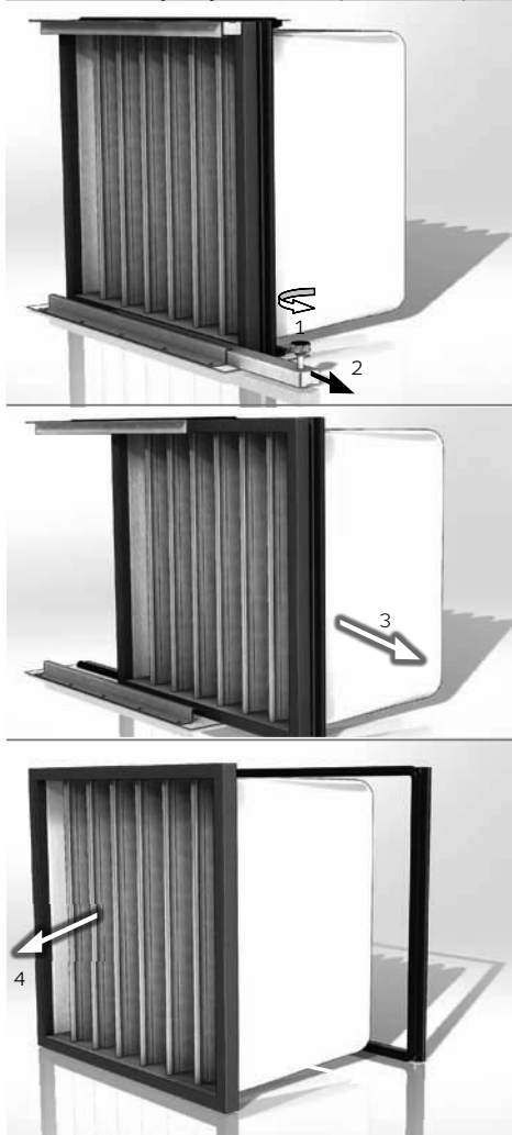
Obrázek 5 – postup vyjmutí filtrační vložky s výsuvným rámečkem (XP04 – XP10)
