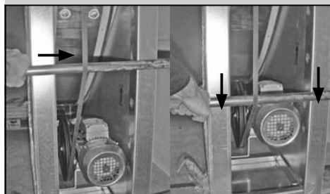
Obrázek 11 – nasazení řemene
