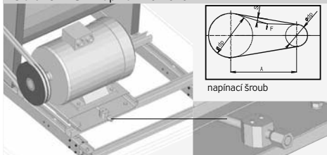
Obrázek 23 – napínání řemene
