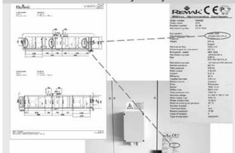
Obrázek 8 – identifikace částí jednotky
