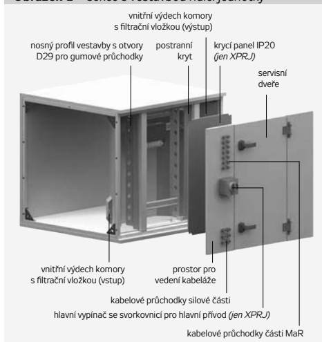
Obrázek 1 – sekce s vestavbou řídicí jednotky
