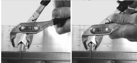
Obrázek 12 – zakrytí a zajištění spoje stříšek
