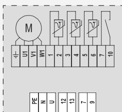
Obrázek 4 – Schéma zapojení rekuperátoru
