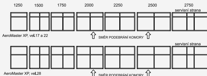
Obrázek 4 – zobrazení podstavných rámu
