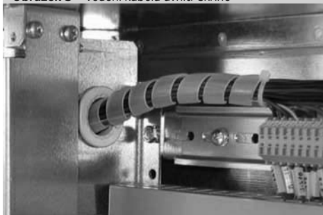
Obrázek 5 – vedení kabelů uvnitř skříně
