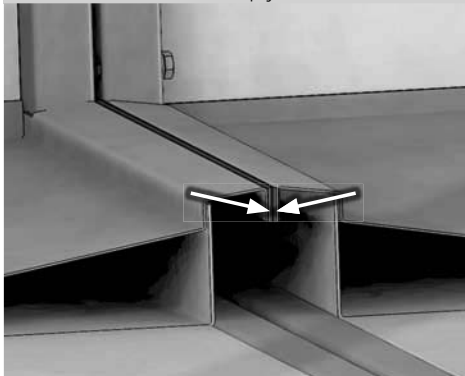
Obrázek 3 – těsnění v místě napojení van
