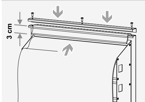
Obrázek 3 – zavedení nové tkaniny
