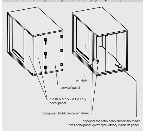
Obrázek 19 – výměníky v sekci s krytými přívody
