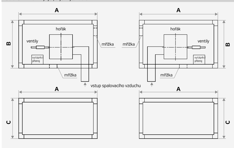
Obrázek 1 – rozměry vytápěných krytů hořáků
