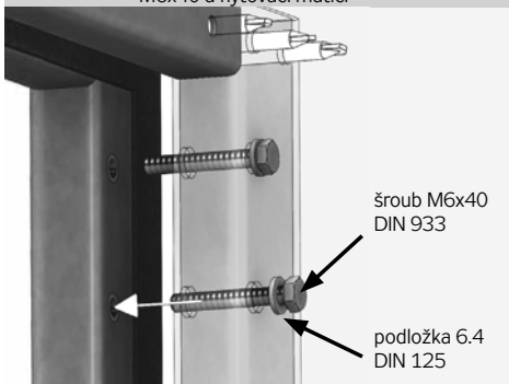
Obrázek 2 – spojení spojovacího rámečku šroubem M6x40 a nýtovací maticí
