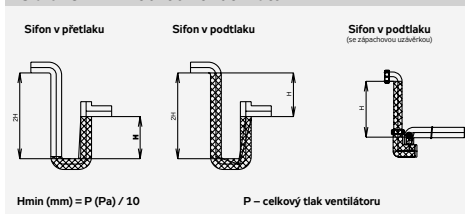
Obrázek 21 – odvod kondenzátu
