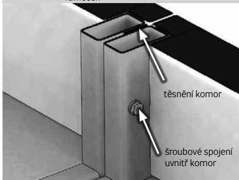
Obrázek 1 – způsob spojení komor přes spojovací rámeček
