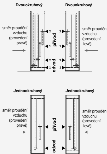
Obrázek 20 – zapojení výparníků
