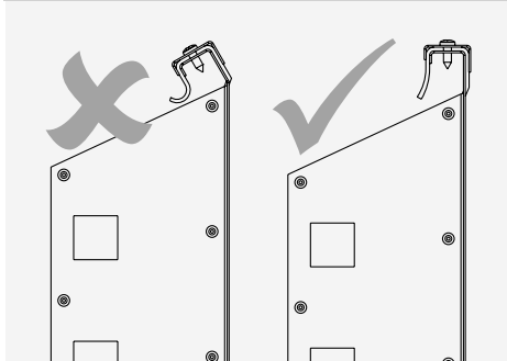
Obrázek 5 – kontrola správnosti montáže
