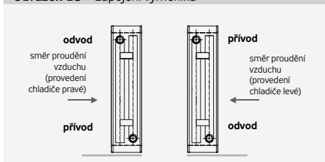
Obrázek 18 – zapojení výměníků
