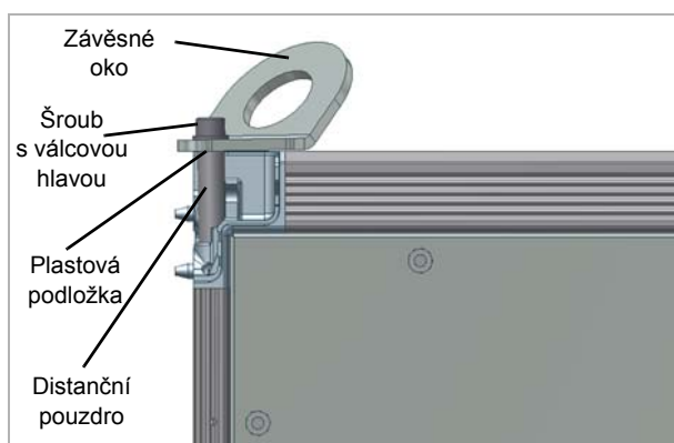
Obr. 5-9: Závěsná oka v transportním dělení
