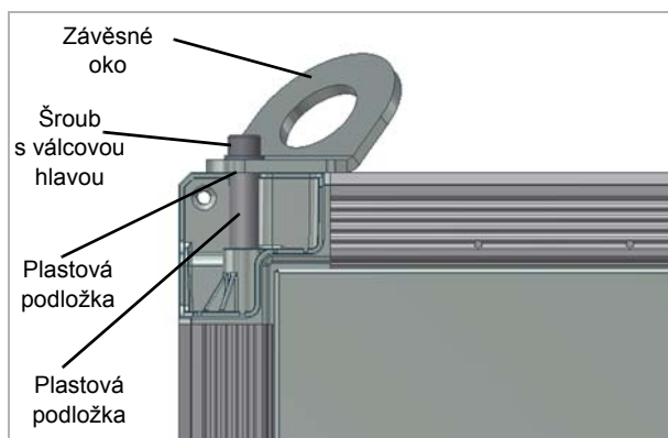
Obr. 5-10: Závěsná oka pro střechu a čelní panel
