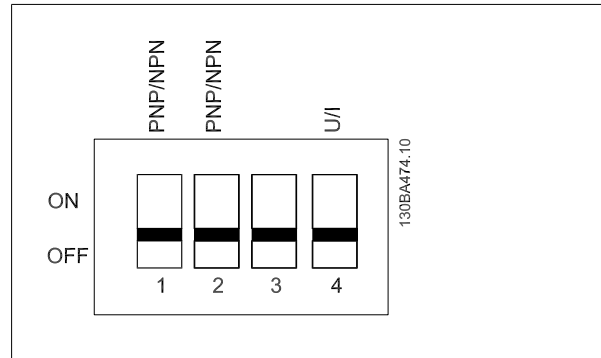
Obrázek 3.9: S200 Přepínače 1-4.
