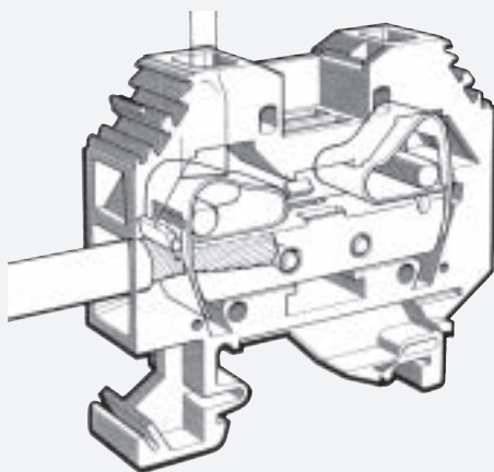
Obrázek 14 – svorka typu WAGO
