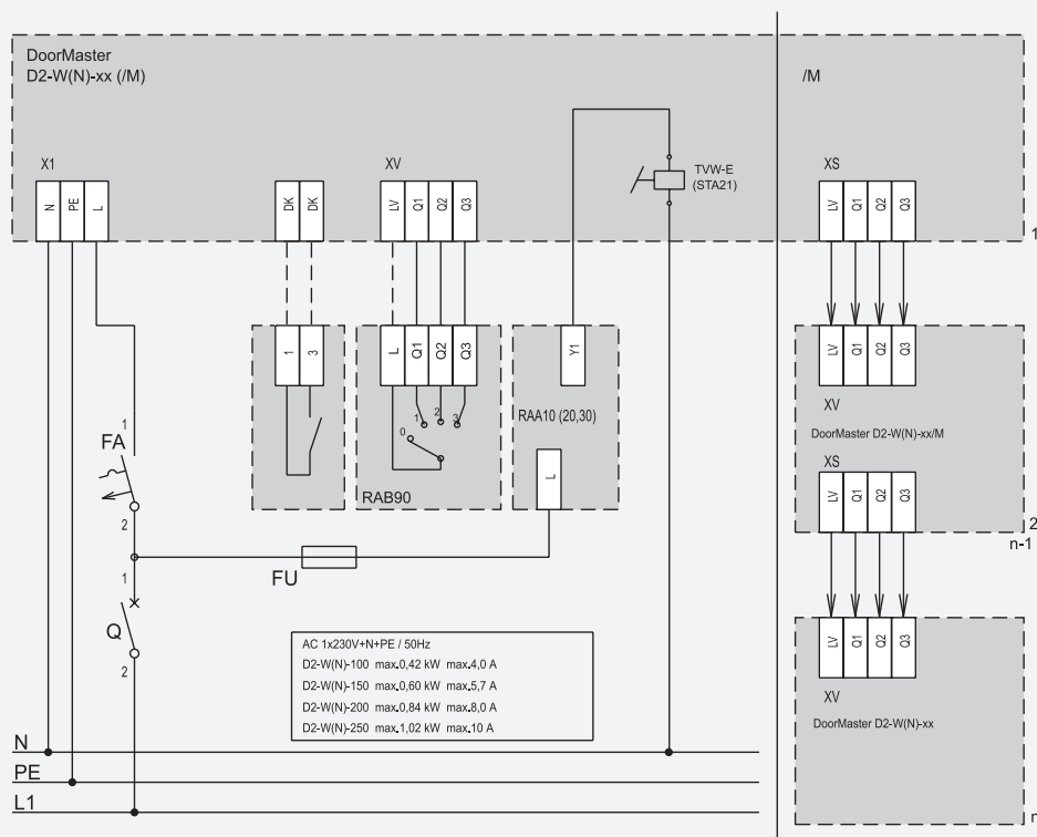
Obrázek 29 – napojení clony D2-W a clony D2-N
