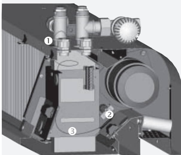
Obrázek 16 – montáž tykavky termostatu, clona C1
