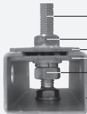
Obrázek 5 – zavěšovací profil
