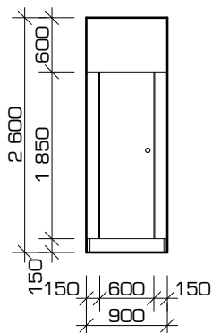
pohled
