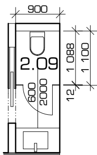
půdorys
