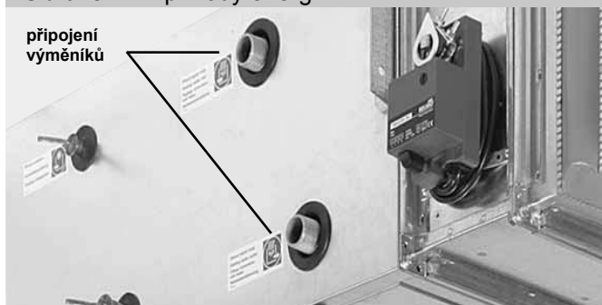
Obrázek 7 – přívody energií
