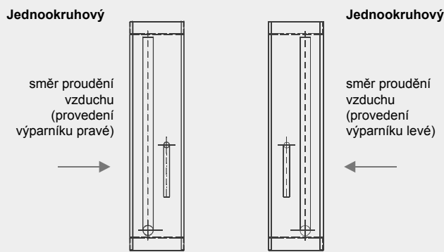
Obrázek 9 – zapojení výparníků
