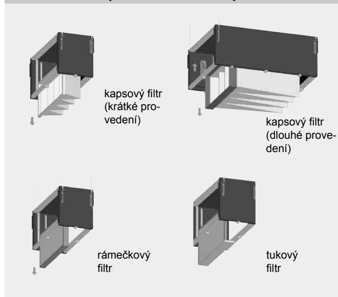
Obrázek 15 – výměna filtrační vložky
