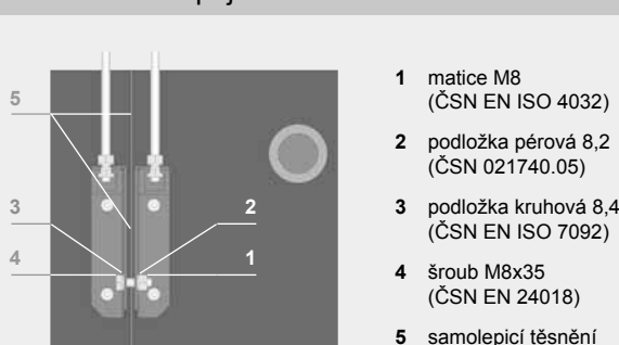
Obrázek 5 – spojení sekcí
