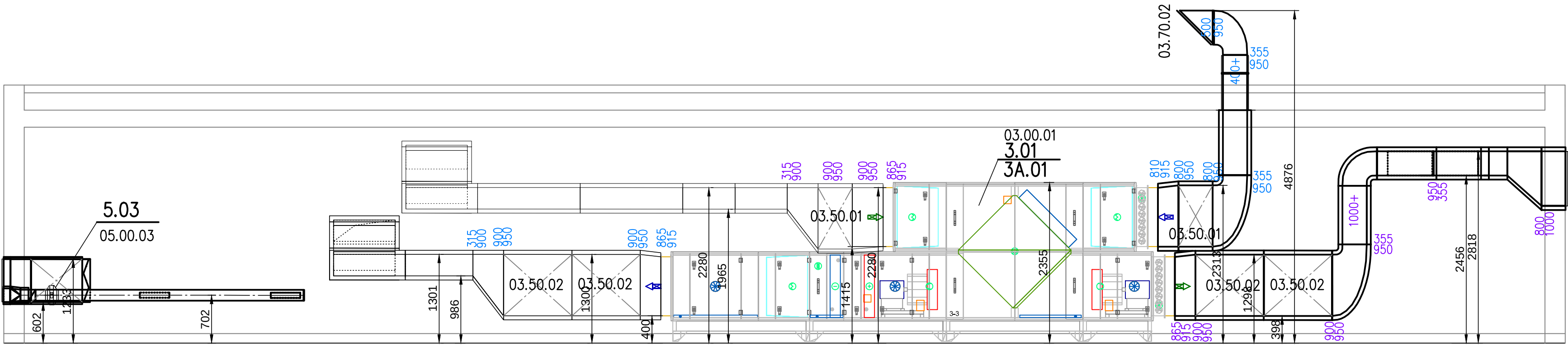
ŘEZ AHU 3-3
