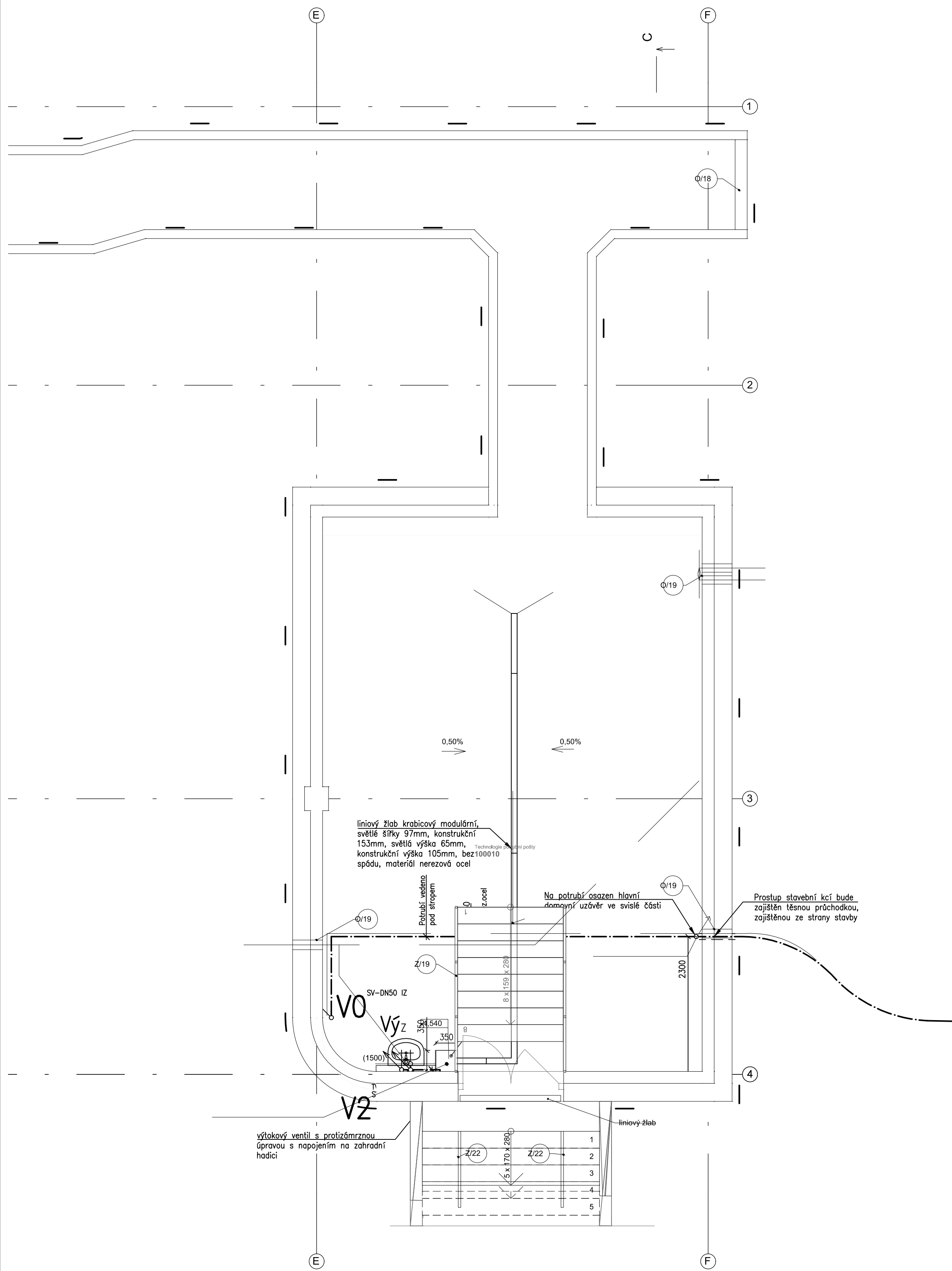
Potrubí teplé vody (TV)
