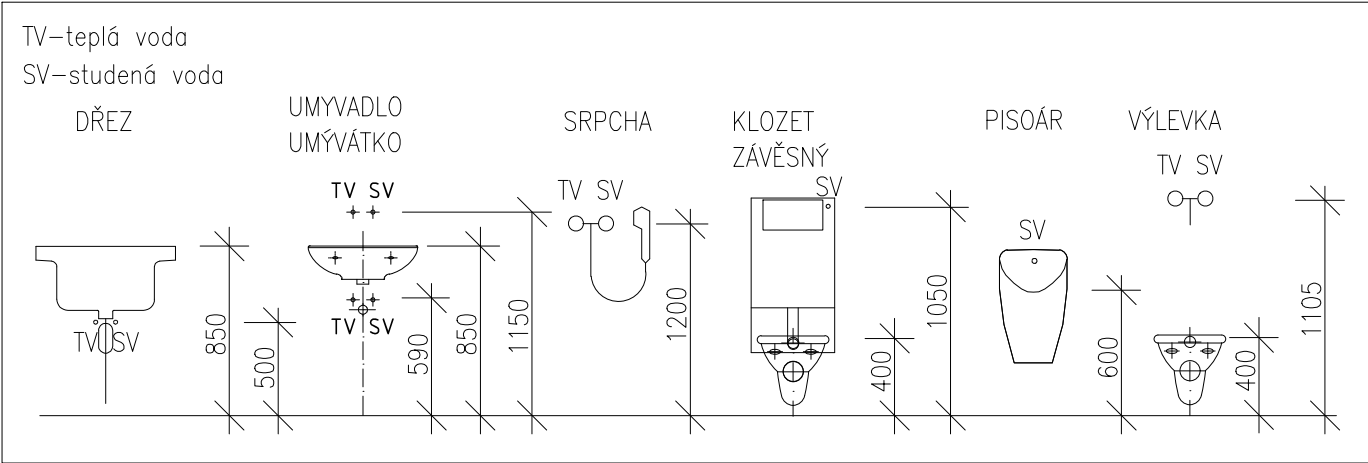
Potrubí teplé vody (TV)
