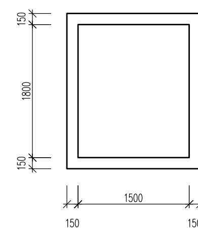
ŘEZ CHRÁNIČKOU POTRUBNÍ POŠTY – 45,0 BM
