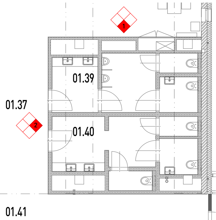
půdorys
