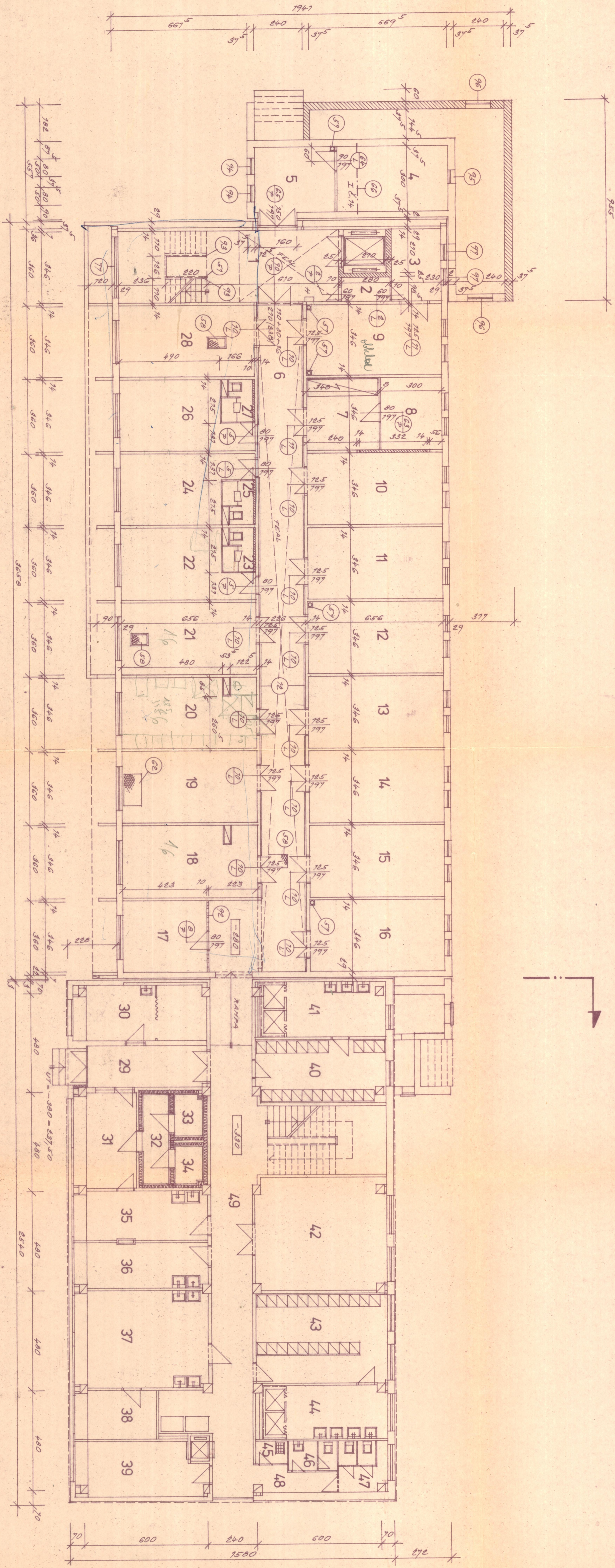
KREVNI BANKA VIX SAMOSTATNY VYKRES 1:50
