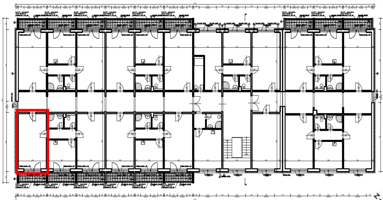
Obrázek 35 - Lokalizace vybrané „kritické místnosti“
