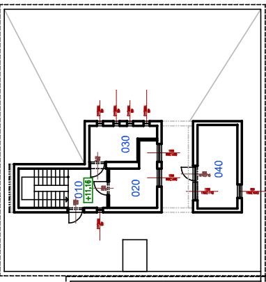
Budova J2 Púdroys 4NP
