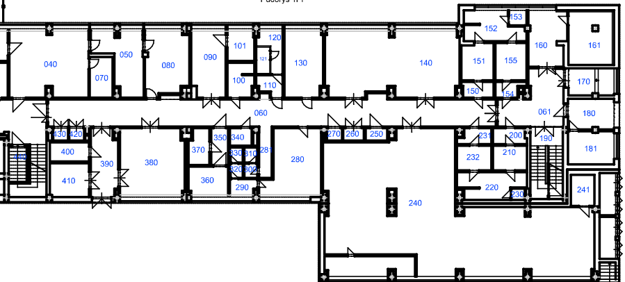
Budova Q2 Púdorys 1PP
